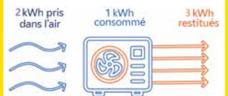
Pompe à chaleur avec un COP égal à trois
